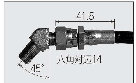
45°エルボ形
