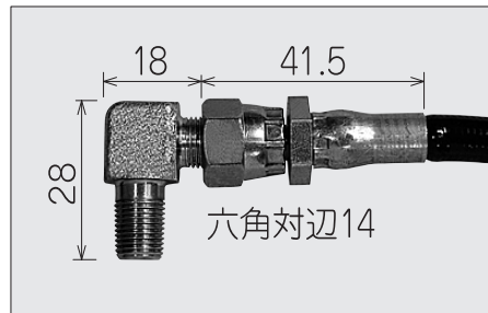
エルボ形
